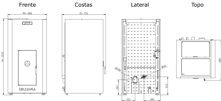
Figura 2 - Dimensões das caldeiras compactas 18 kW e 24 kW
