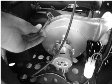
Figura 33 - a) Retirar os parafusos; b) Retirar extractor
