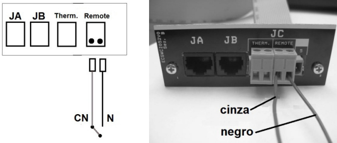
Figura 20 - Ligações do comando externo com fios
