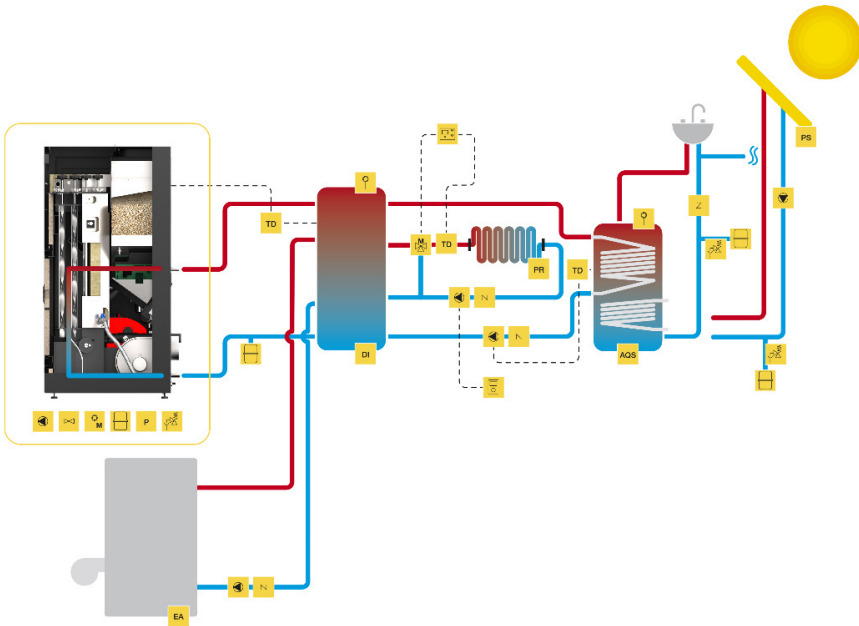
Figura 40 - Ligação a chão radiante, conjugado com outra caldeira de apoio e águas sanitárias combinado com painel solar
