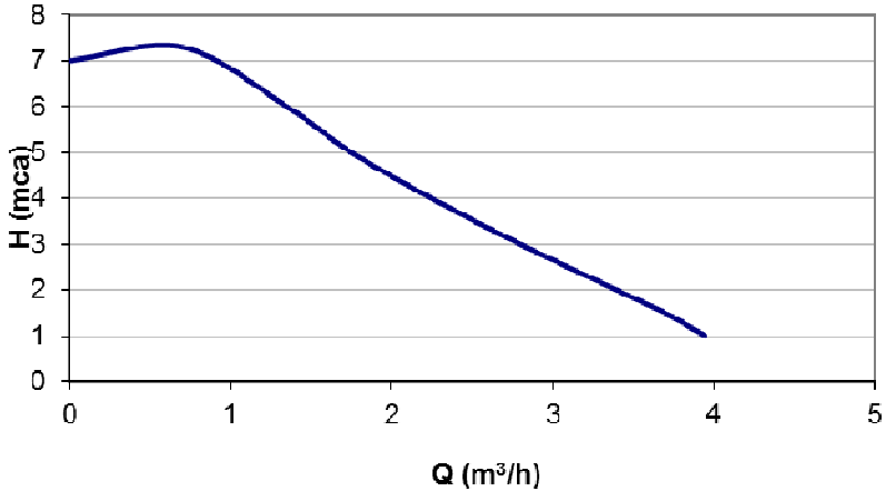
Figura 44 - Gráfico de desempenho da bomba
