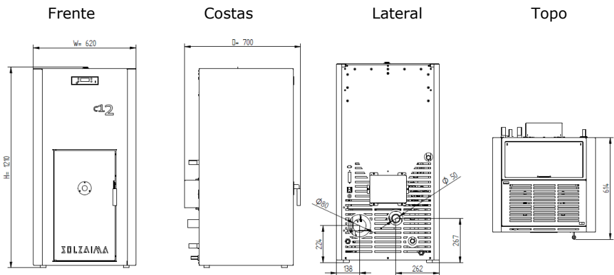
Figura 4 - Dimensões da caldeira compacta 12 kW
