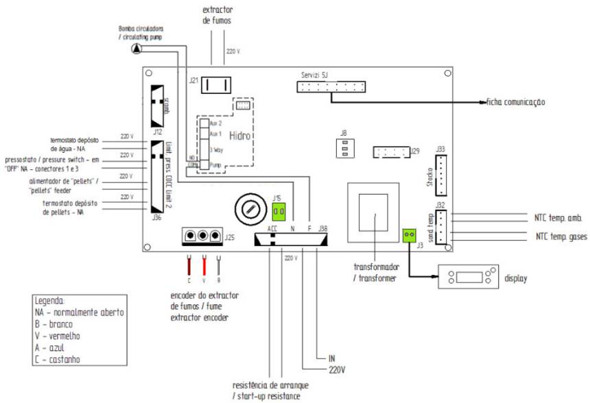
Figura 42 - Esquema eléctrico Compacta 12 kW
